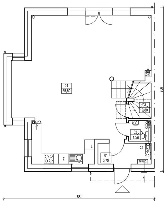
PARTER - 61,60 M 2
