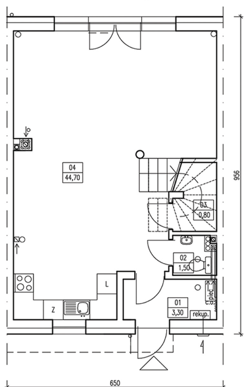
PARTER - 50,30 M 2
